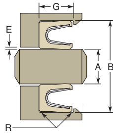
Rod Seal
