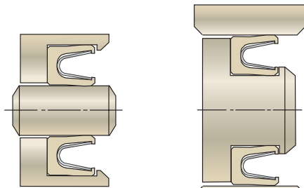
Rod Gland
