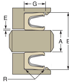
Rod Seal
