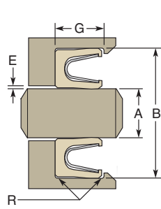
Rod Seal
