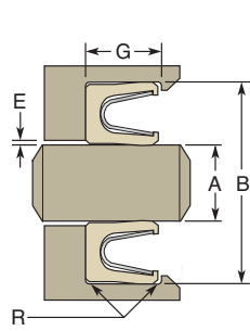
Rod Seal
