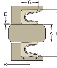
Rod Seal
